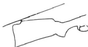
Monte Carlo
