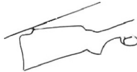
Monte Carlo
